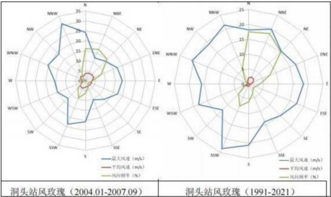
洞头气象站风玫瑰图
